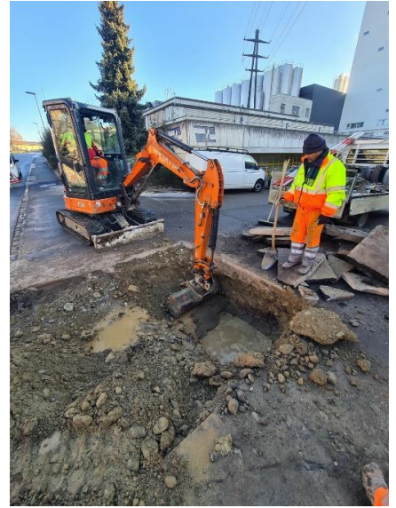
1b. Excavation sur la conduite
