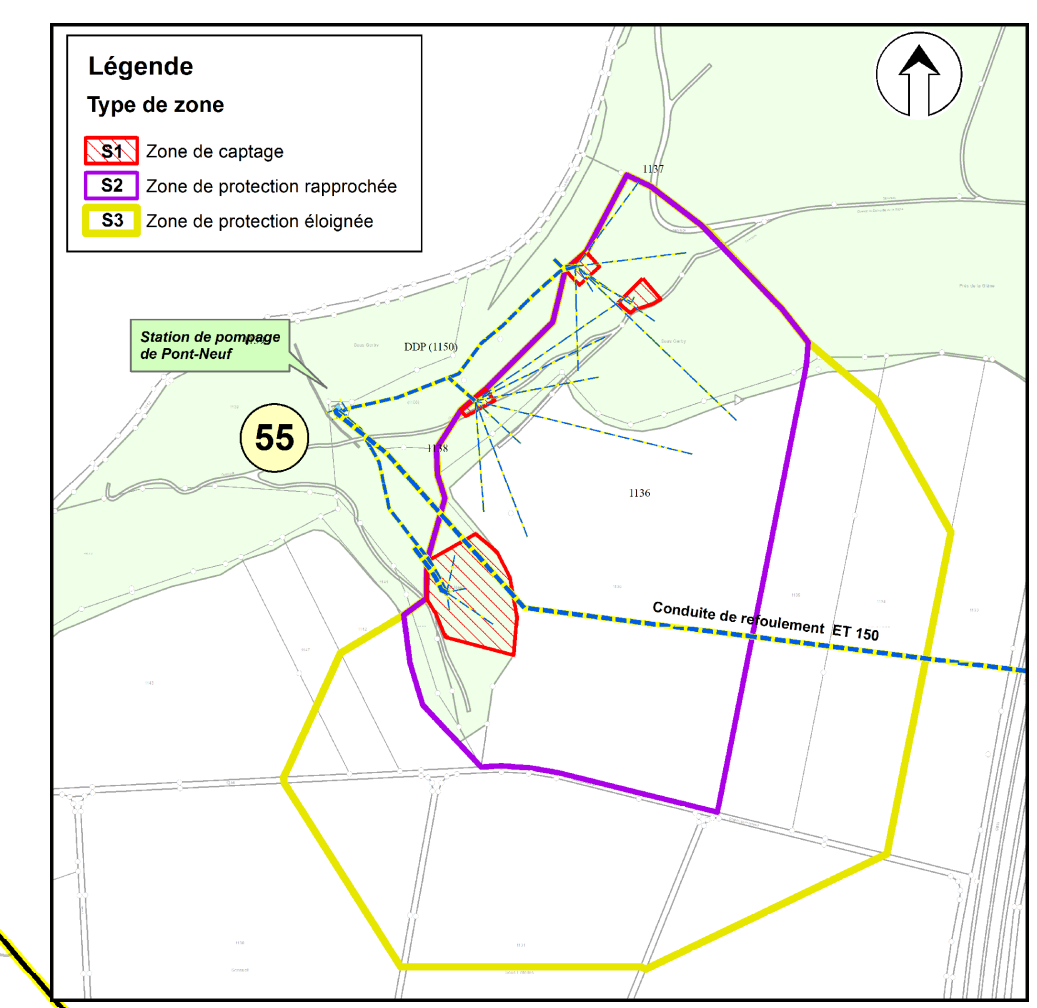
Commune de Hauterive FR Captage de Pont-Neuf
